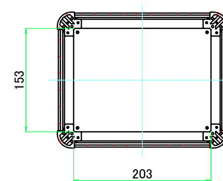
C-C ( 1 : 5.5 )
